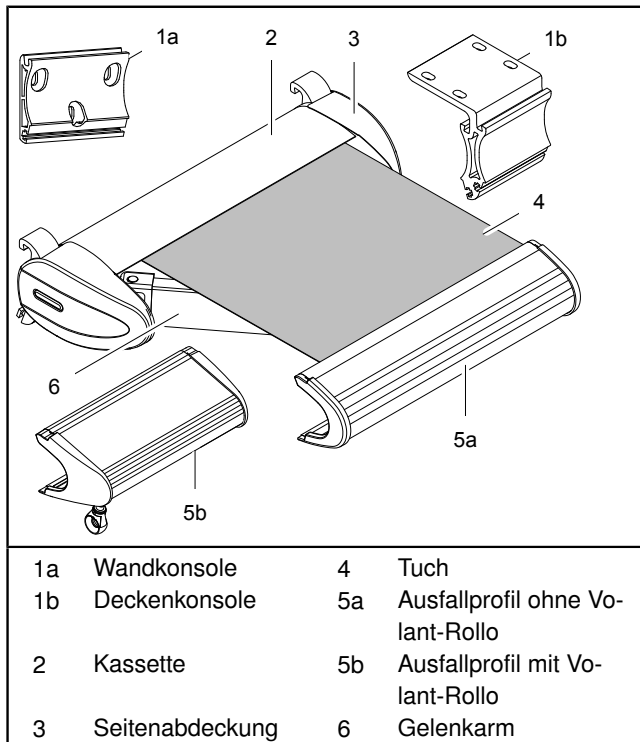
Abb. 1: Teileübersicht Kassetten-Markise Typ 580
