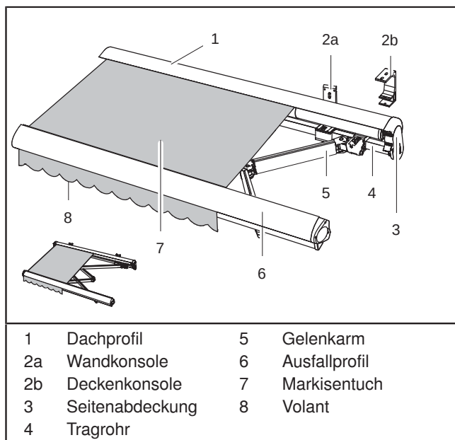
Abb. 1: Teileübersicht Gelenkarm-Markise Typ 750
