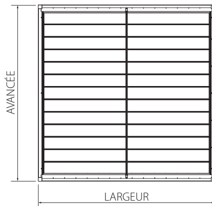
3 GLISSIÈRES MODULE SIMPLE Vue du dessus
